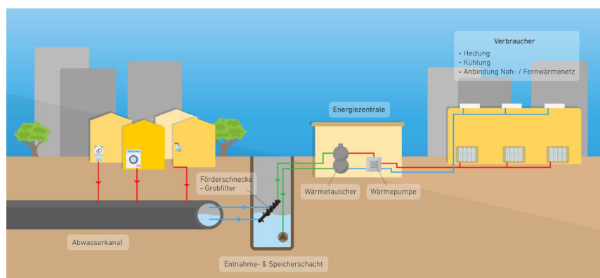
Schema 4: Nutzung Kanalabwasserwärme mit extern angebrachten Wärmetauschern
