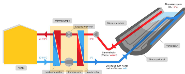
Schema 3: Nutzung Kanalabwasserwärme mit im Kanal eingebauten Wärmetauschersystemen
